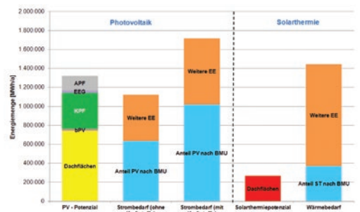
Potenzialauswertung Gesamtpotenzial für die Stadt und den Landkreis Bamberg [MWh/a]
