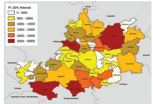
Darstellung Freiflächenpotenzial Photovoltaik je Gemeinde [MWh el /a]
