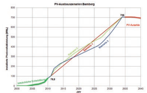
Darstellung PV-Ausbauszenarien
