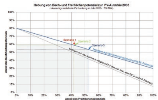
Abhängigkeit der Ausbaurrate von Dach- und Freifläche
