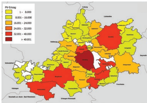
Darstellung Dachflächenpotenzial Photovoltaik je Gemeinde [MWh el /a]
