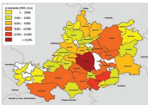
Darstellung Dachflächenpotenzial Solarthermie je Gemeinde [MWh th /a]
